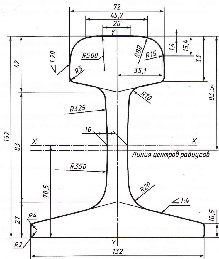
Рисунок А.1 — Рельс типа Р50
